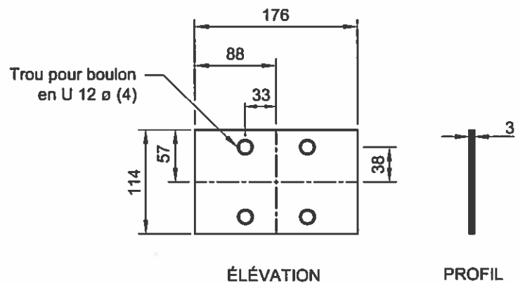
DÉTAIL DE LA PLAQUE ANTIROTATION
